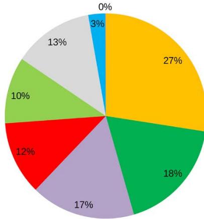
Graphique 15 : Polluants identifiés dans les sols ou les nappes des sites et sols pollués
