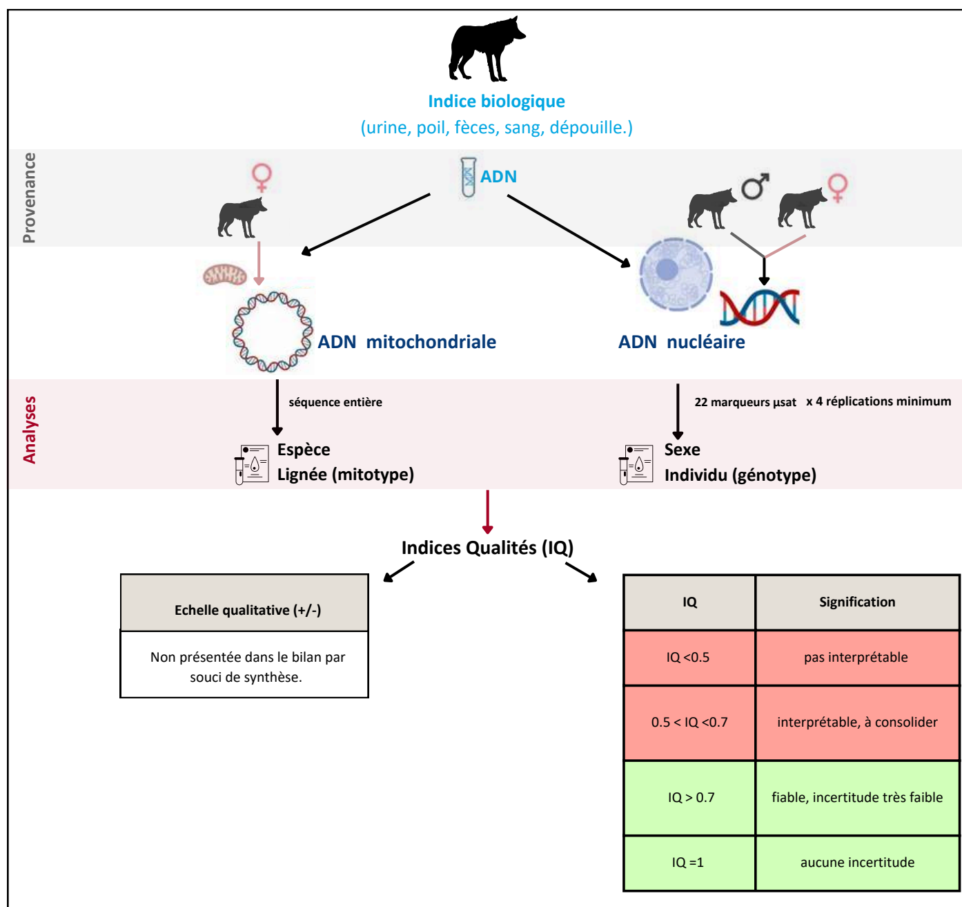
Figure 1 : méthode des analyses génétiques effectuées dans le cadre du suivi de la population lupine française. Deux sources d'ADN différentes sont utilisées afin d'obtenir différents types d'informations (espèce, lignée, sexe, génotype) et de nous permettre d'avoir le profil génétique le plus complet possible pour chaque échantillon.
