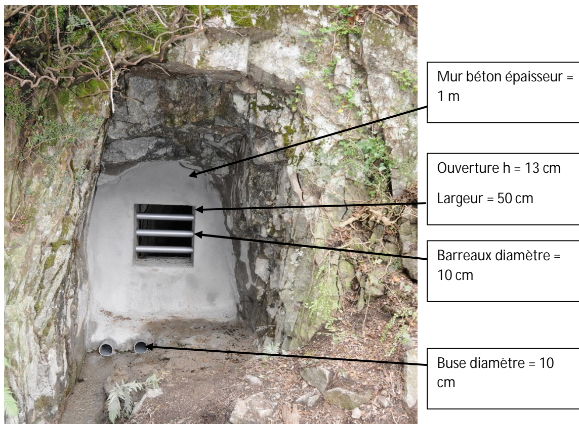
Figure 30 : Exemple de galerie condamnée par un mur en béton, avec passage chiroptère et passage faune rampante aménagé.
