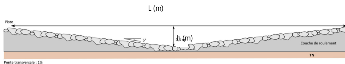
Figure 14 : Dimensionnement des radiers
