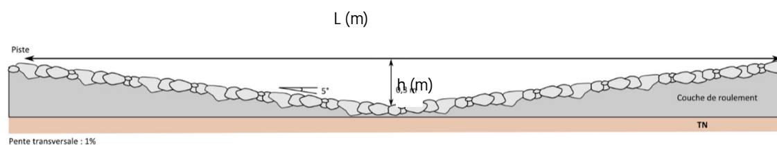
Figure 13 : Dimensionnement des radiers
