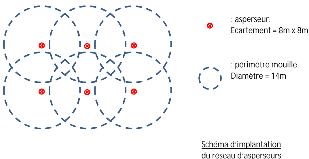
Figure 10 : Exemple d'irrigation par aspersion pouvant être mise en place sur le site des Avinières.
