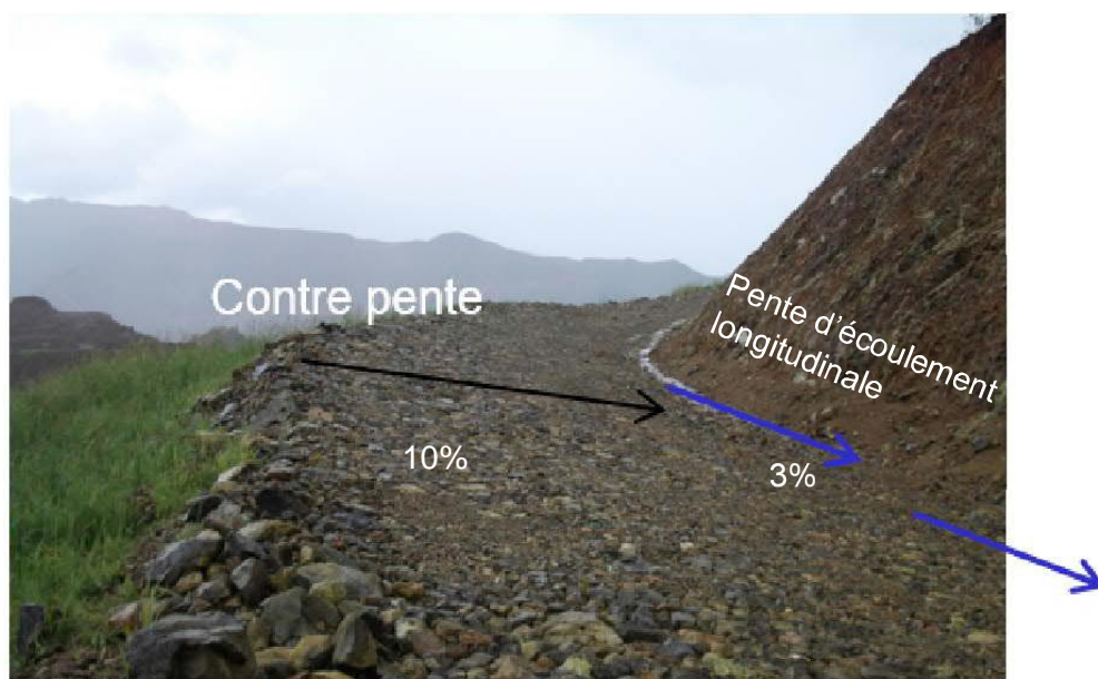
Figure 26 : Exemple de banquette drainante.
