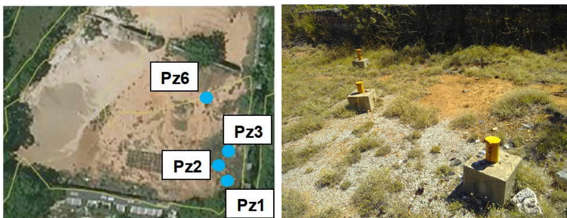
Figure 19 : Emplacement et photographie des piézomètres du bassin à résidus n°1 à conserver et rehausser.
