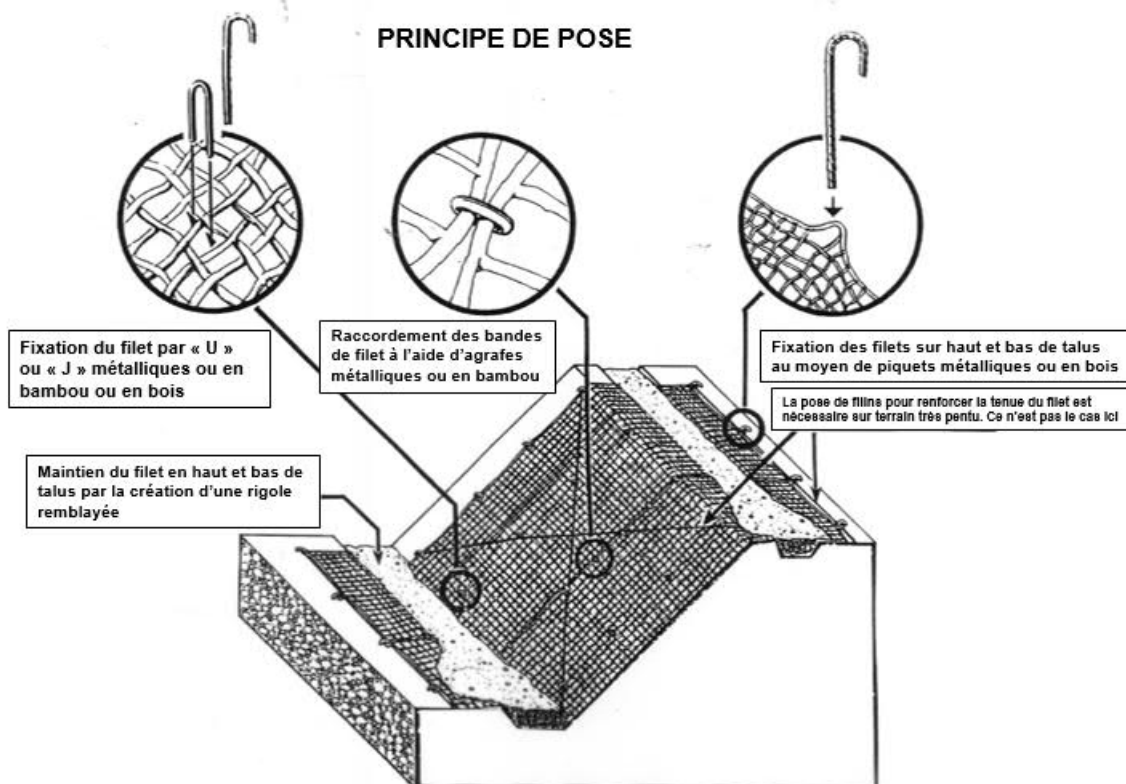
Figure 23 : Principe de pose du géofilet en fibres de coco
