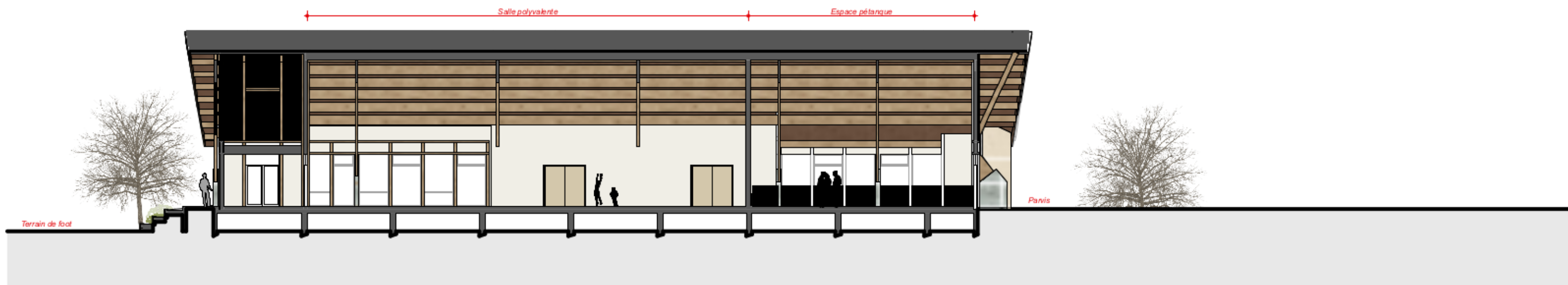
COUPE LONGITUDINALE Ech 1/200°
