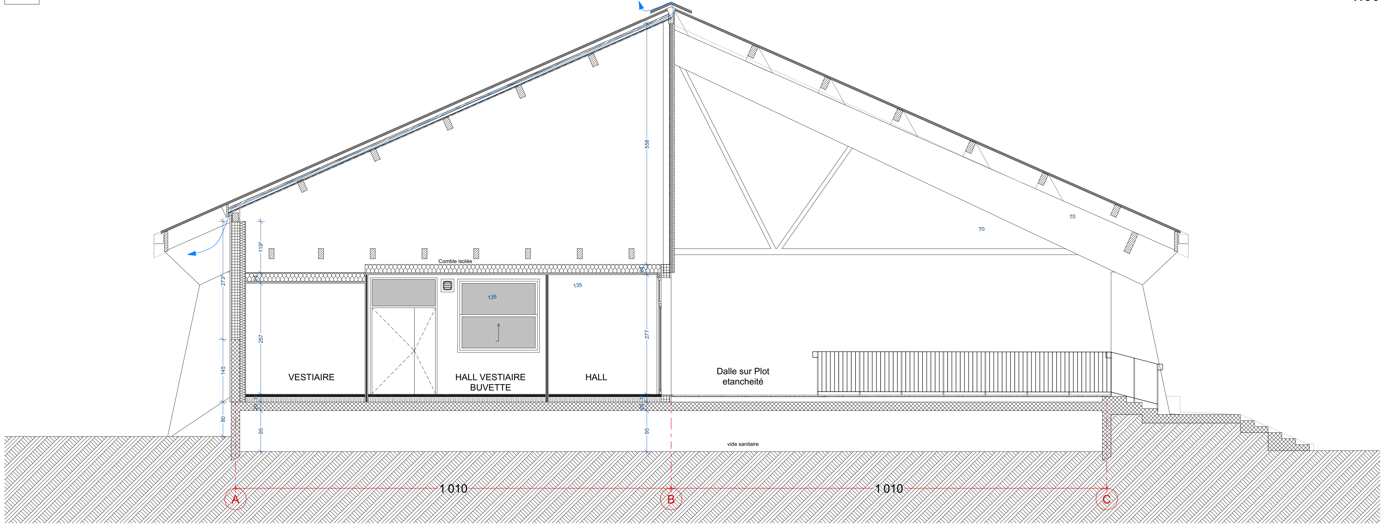
COUPE T13
