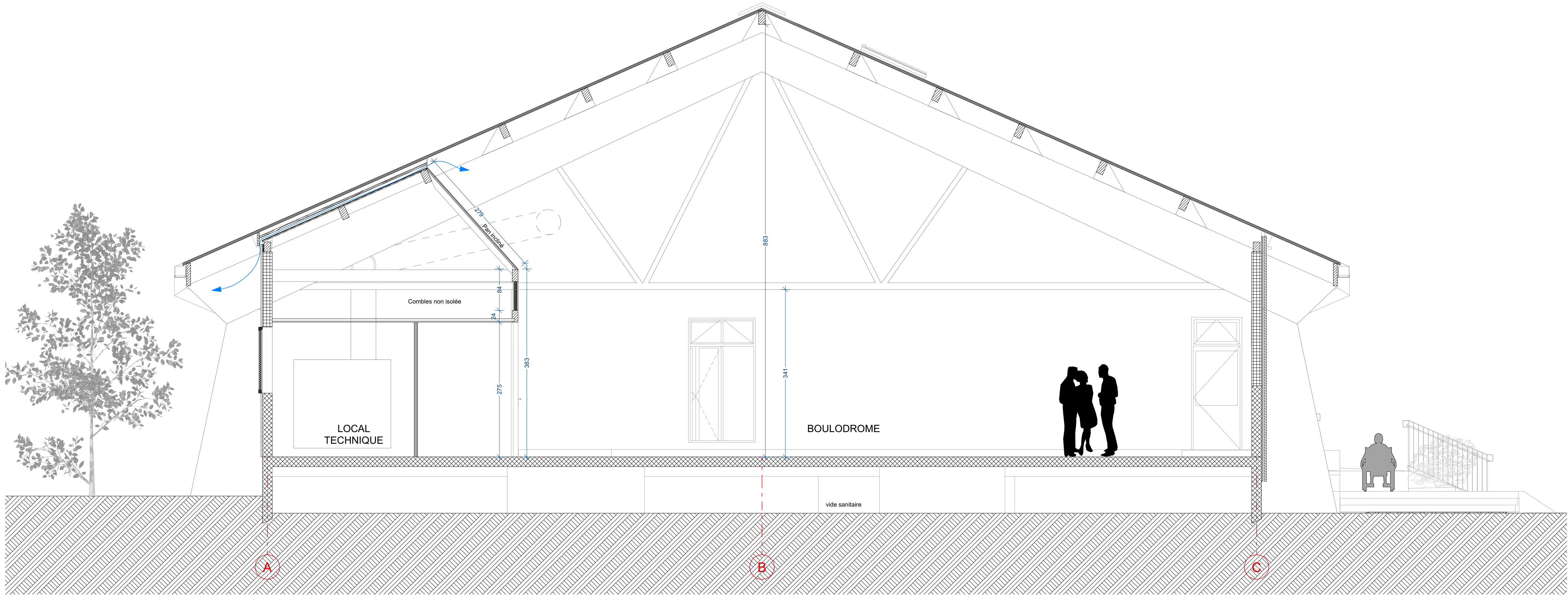
COUPE T2
