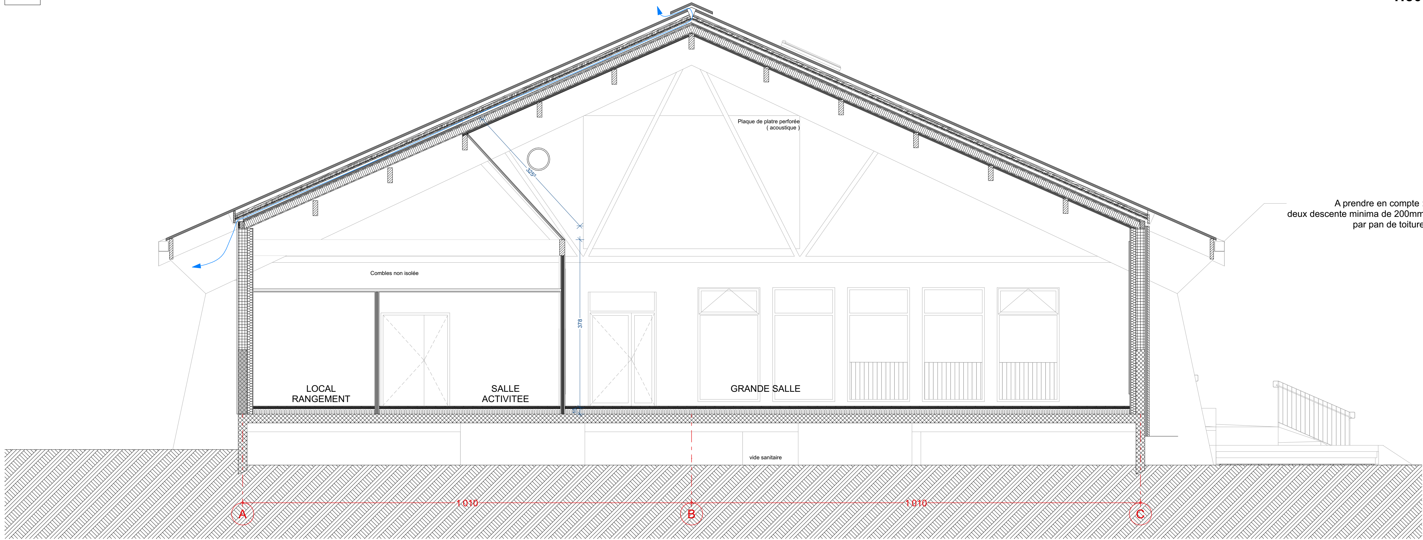
COUPE T8
