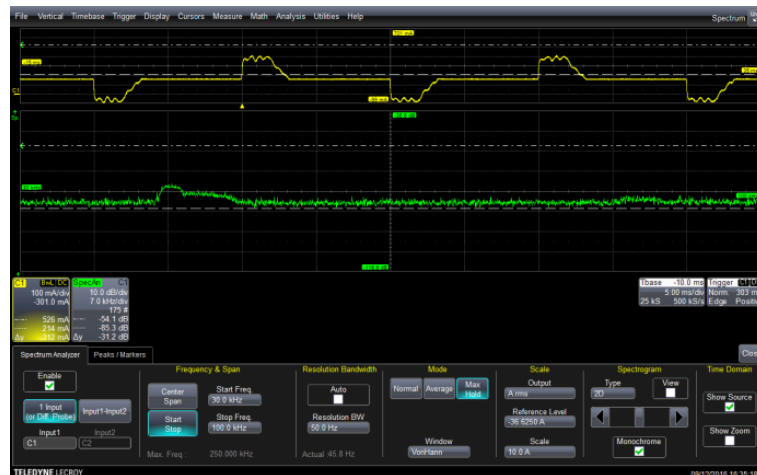
Figure 5-8: courant électrique (en haut) et spectre dans la bande 30 kHz – 95 kHz (en bas) Câble branché sur une lampe fluo compacte
